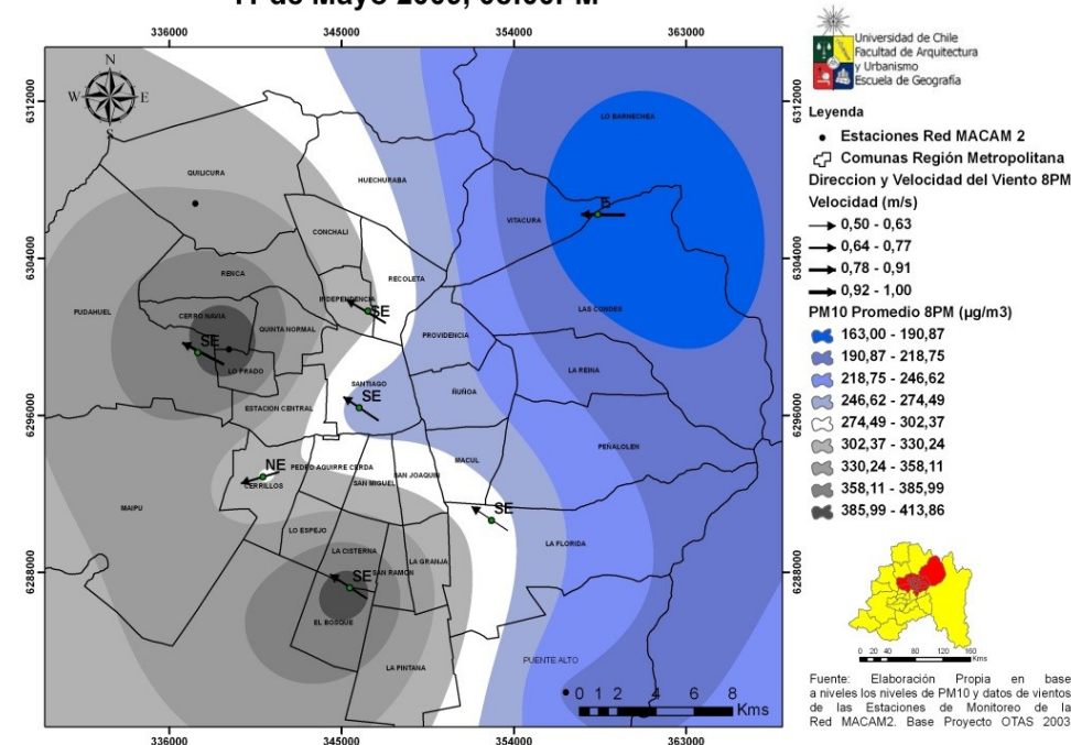
Contaminación por PM10 y Vientos en Santiago 11 de Mayo 2009, 08:00PM
